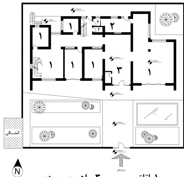
تصویر ۲۰. پلان همکف خانه شماره ۵ با مقیاس ۱/۲۵۰. مأخذ: نگارندگان.
