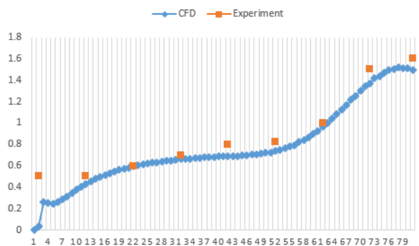
تصویر ۸. تطبیق نتایج برداشت میدانی و داده‌های CFD در ارتباط با شاخص سرعت هوا در حیاط خانه گلشن. مأخذ: نگارندگان.
