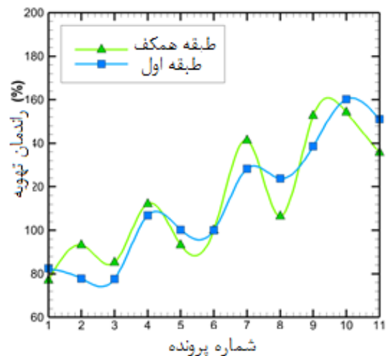
تصویر ۱۵. مقادیر راندمان تهویه برای هر کدام از اتاق های موجود در طبقات همکف و طبقات اول نمونه های موردی. مأخذ: نگارندگان.
