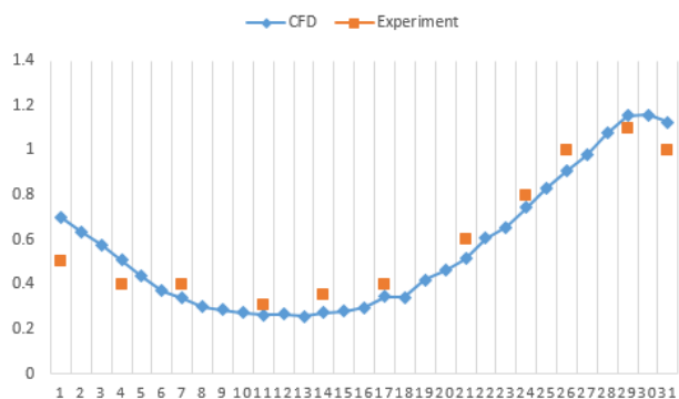
تصویر ۹. تطبیق نتایج برداشت میدانی و داده‌های CFD در ارتباط با شاخص سرعت هوا در اتاق واقع در جبهه شمالی طبقه اول خانه گلشن. مأخذ: نگارندگان.
